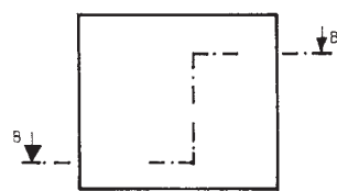
geknickter Schnitt
